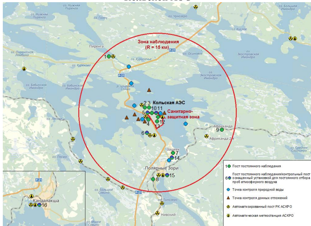
Рисунок 6. Карта-схема проведения радиационного контроля в районе расположения Кольской АЭС
