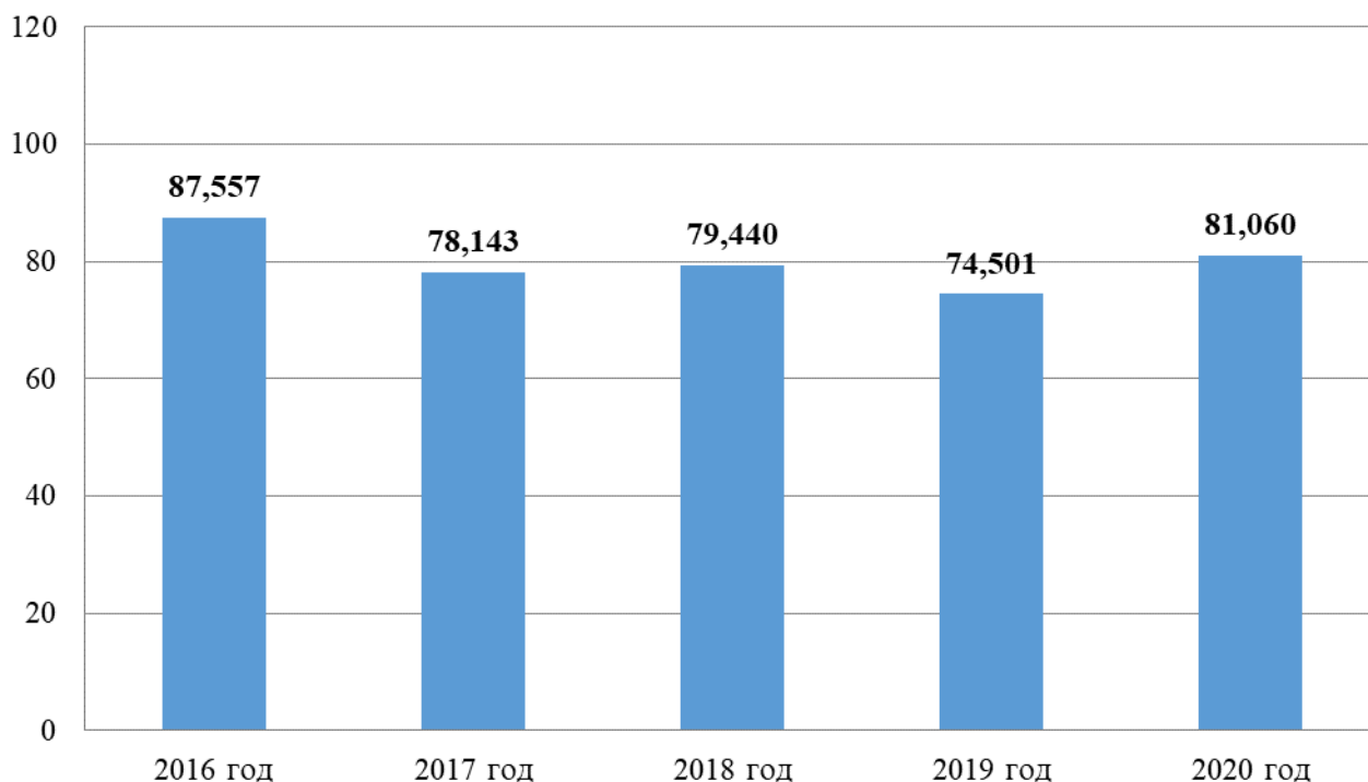
Диаграмма 3. Динамика выбросов загрязняющих веществ в атмосферный воздух, тонн/год
