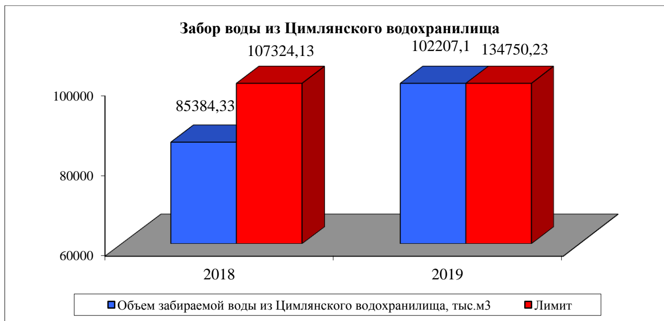
Диаграмма 1. Забор воды из Цимлянского водохранилища за 2018-2019 года
