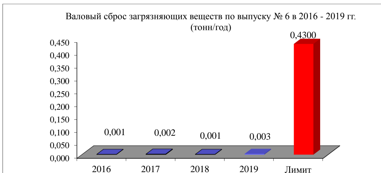
Диаграмма 14. Валовый сброс загрязняющих веществ по выпуску № 6 за 2016-2019 года
