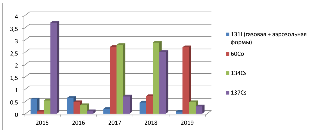
Диаграмма 17. Динамика активности газоаerosольных выбросов Ростовской АЭС за 2015-2019 год (% от ДВ).
