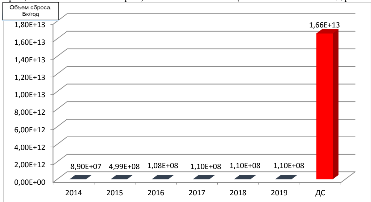
Рис. 4. Сбросы радионуклидов трития в водные объекты Ростовской АЭС, Бк/год
