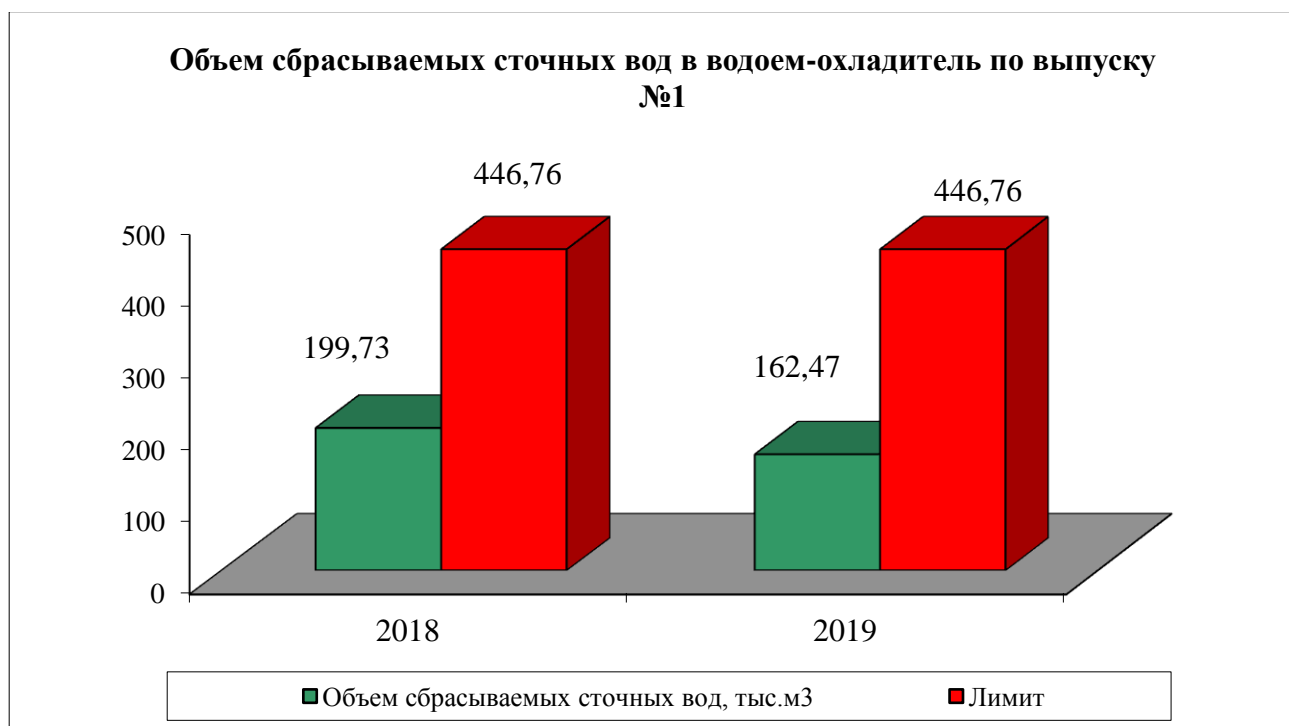
Диаграмма 3. Объем сбрасываемых сточных вод по выпуску №1 за 2018-2019 года
