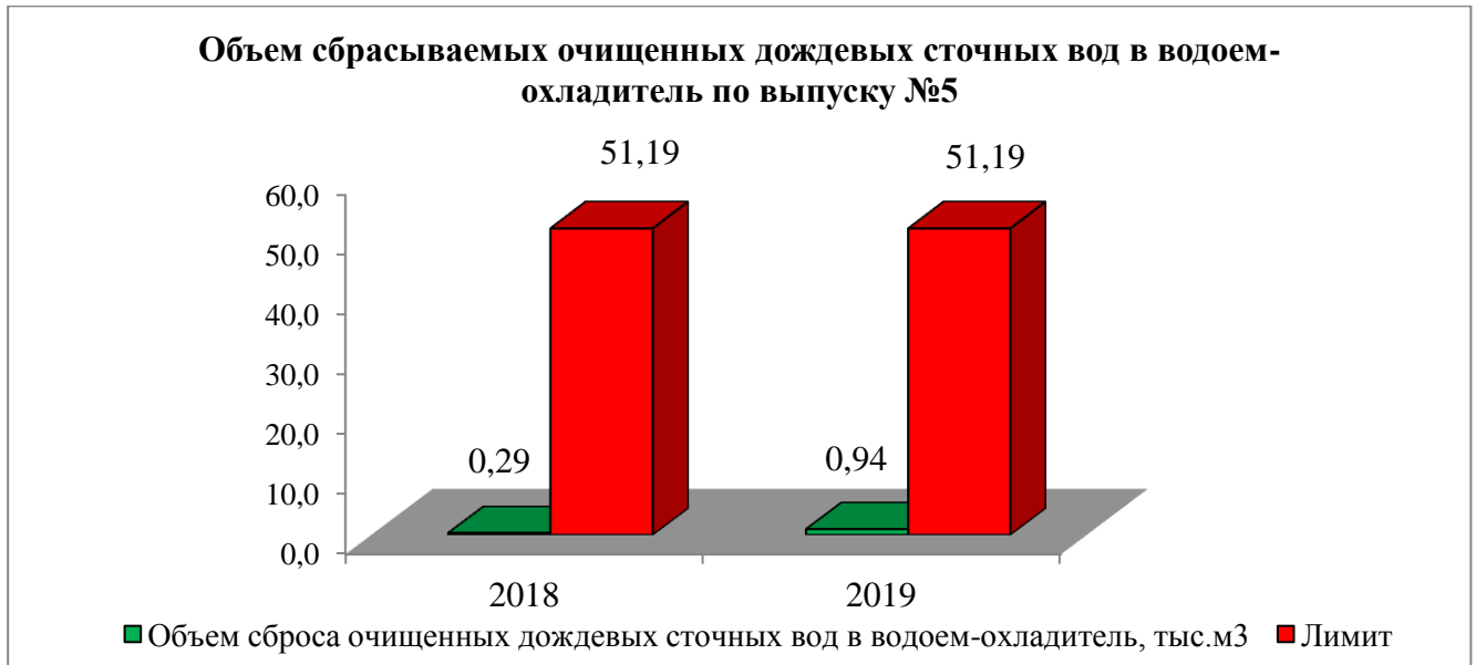
Диаграмма 6. Объем сбрасываемых ливневых вод (выпуск №5) за 2018-2019 года
