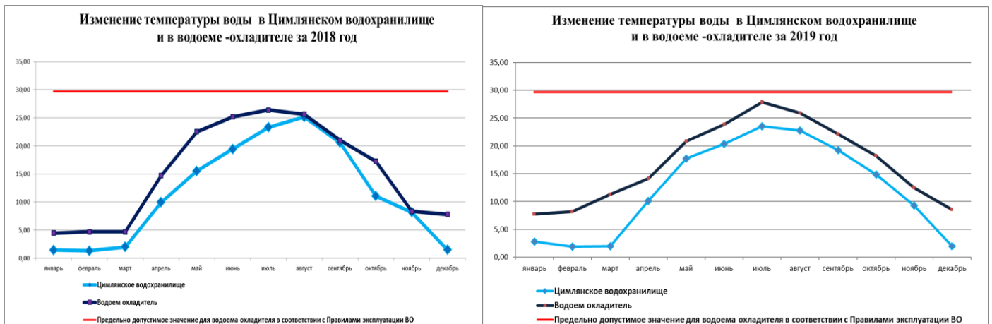
Рис. 3. Результаты мониторинга среднесуточной температуры воды водоема-охладителя и Цимлянского водохранилища в 2018-2019
