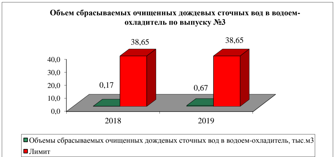
Диаграмма 5. Объем сбрасываемых сточных вод (выпуск №3) за 2018-2019 гг.
