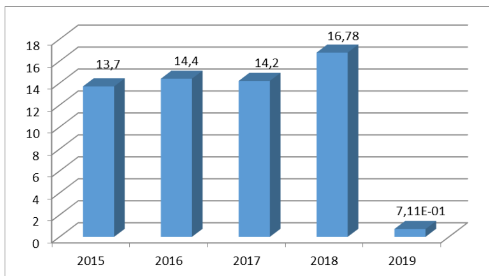
Диаграмма 18. Динамика выброса ИРГ Ростовской АЭС за 2015-2019 года (% от ДВ).
