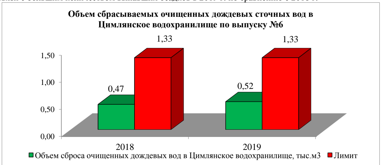
Диаграмма 7. Объем сбрасываемых ливневых вод (выпуск №6) за 2018-2019 года
