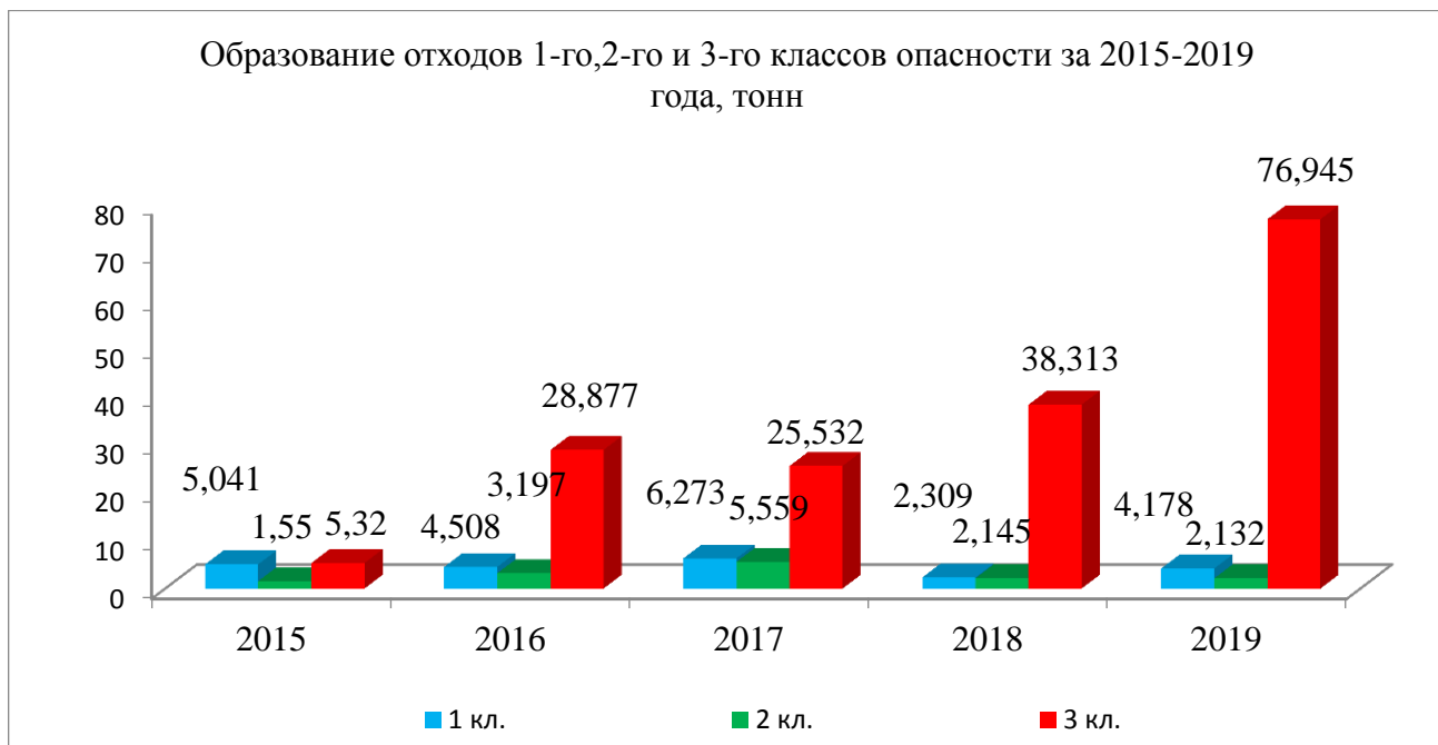
Диаграмма 21. Образование отходов 1,2,3 класса опасности на предприятии за 2015-2019 года
