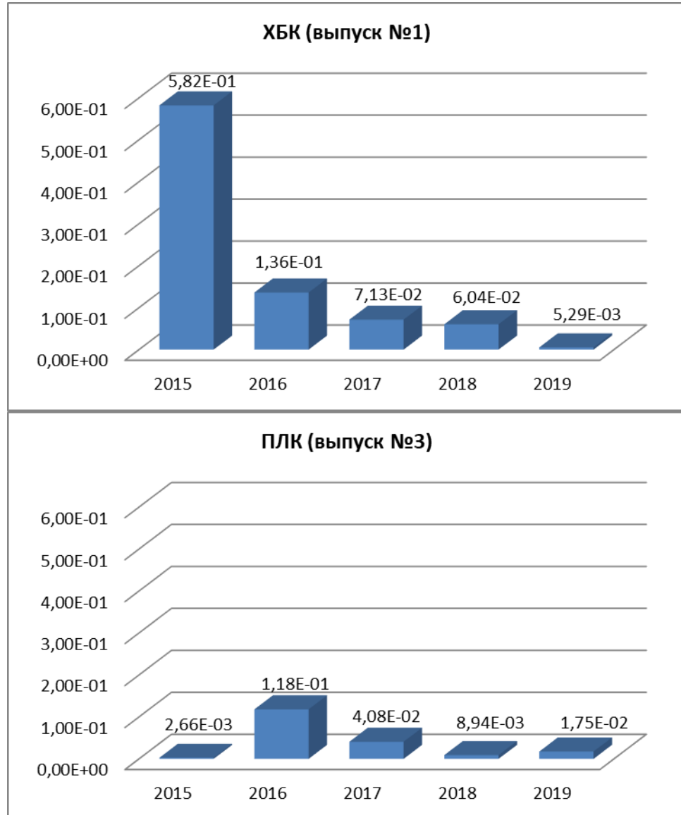
Диаграмма 15. Динамика изменения индекса сброса радионуклидов в водоем-охладитель Ростовской АЭС за 2015-2019 годы
