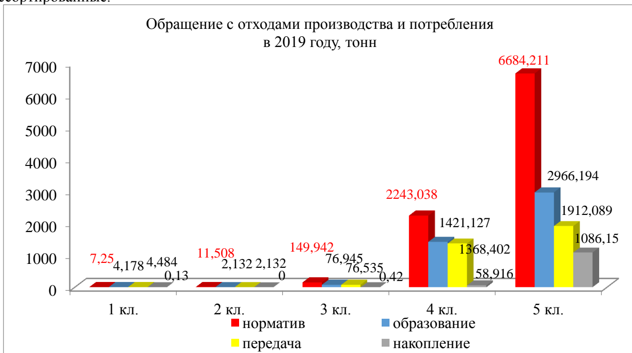
Диаграмма 19. Обращение с отходами производства и потребления в 2019 г.
