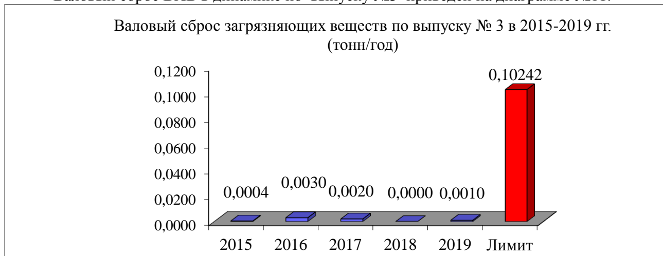
Диаграмма 11. Валовый сброс загрязняющих веществ по выпуску № 3 за 2015-2019 года
