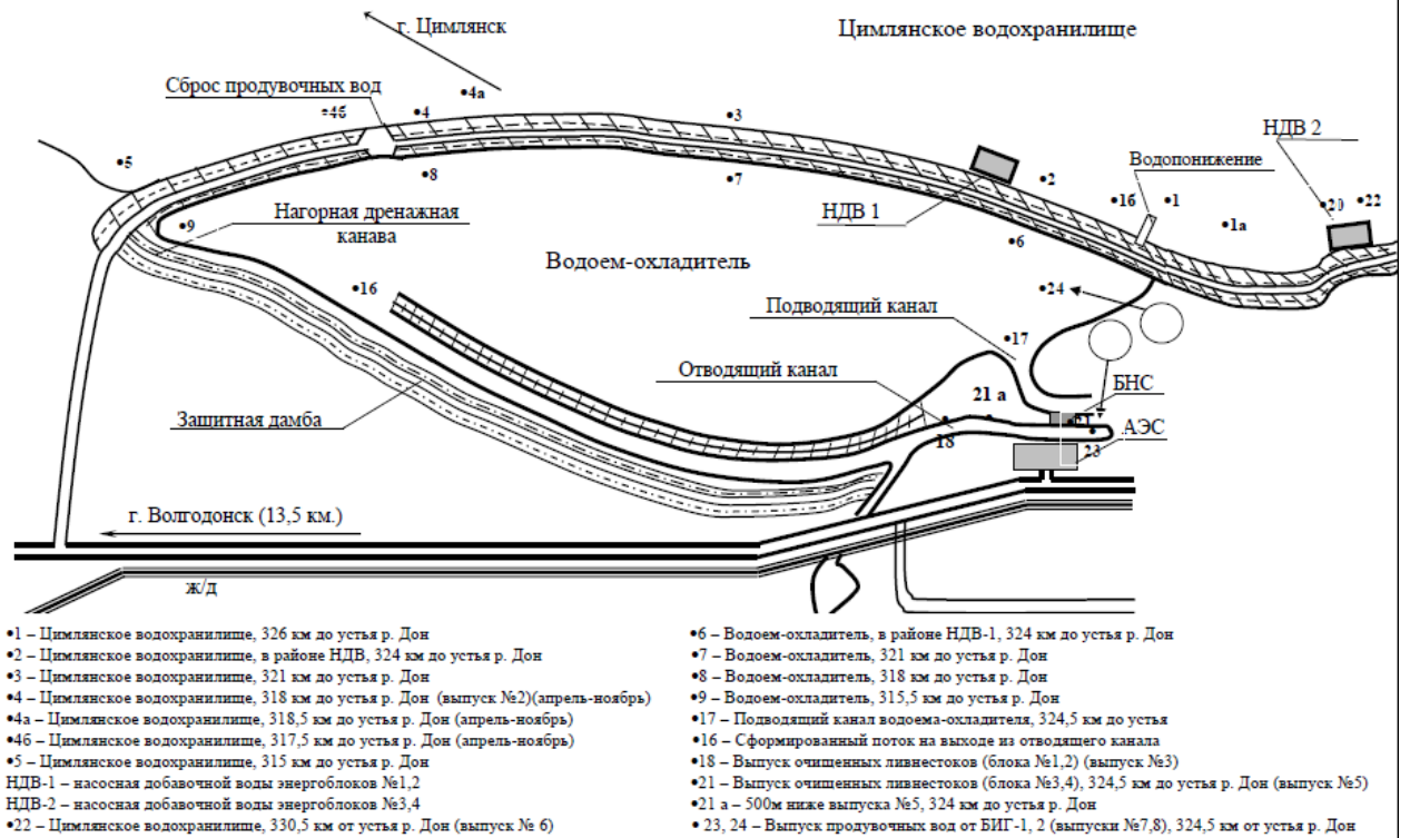
Рис. 1. Схема точек отбора проб ЛООС ООС из Цимлянского водохранилища и водоема-охладителя Ростовской АЭС
