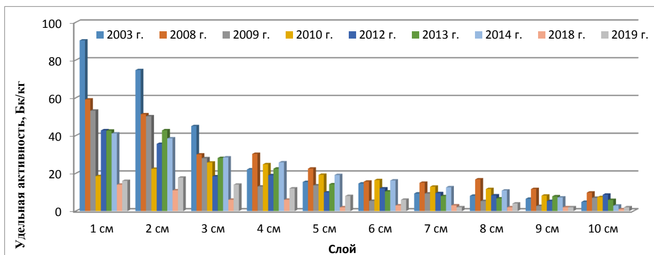
Рис. 6. Результаты мониторинга почвенного покрова уд.активности Cs-137.
