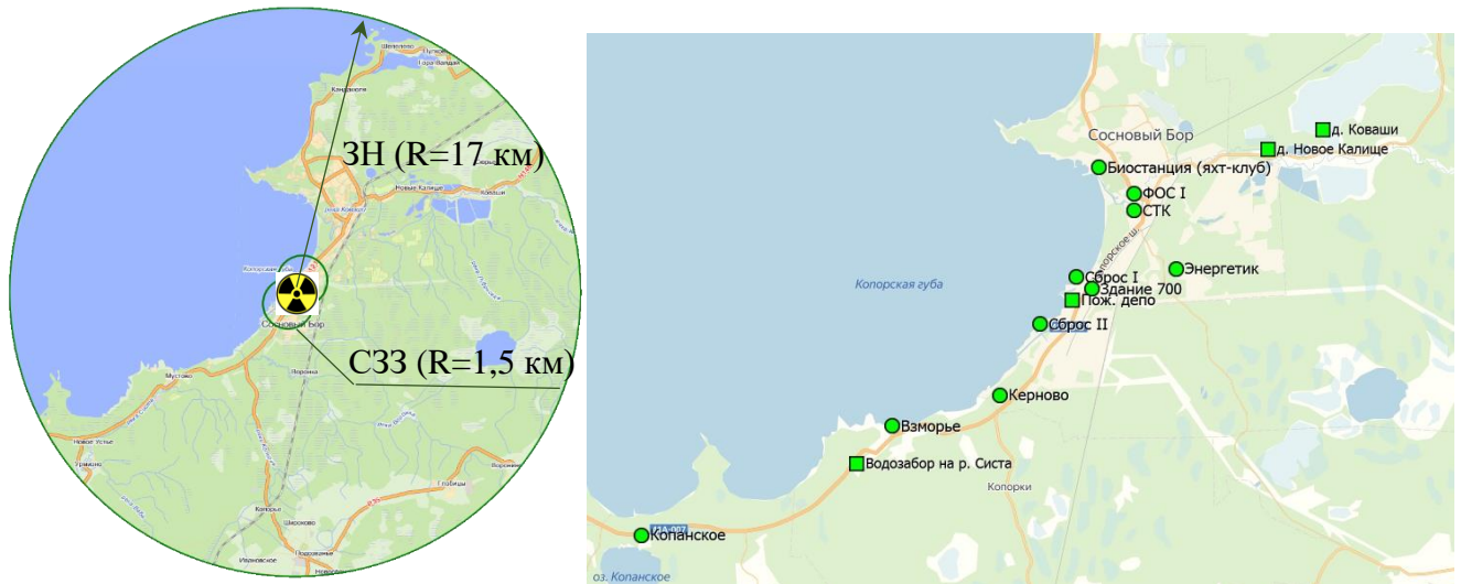
Рис. 5.1. Санитарно-защитная зона и зона наблюдений Ленинградской АЭС, расположение постов модернизированной АСКРО
