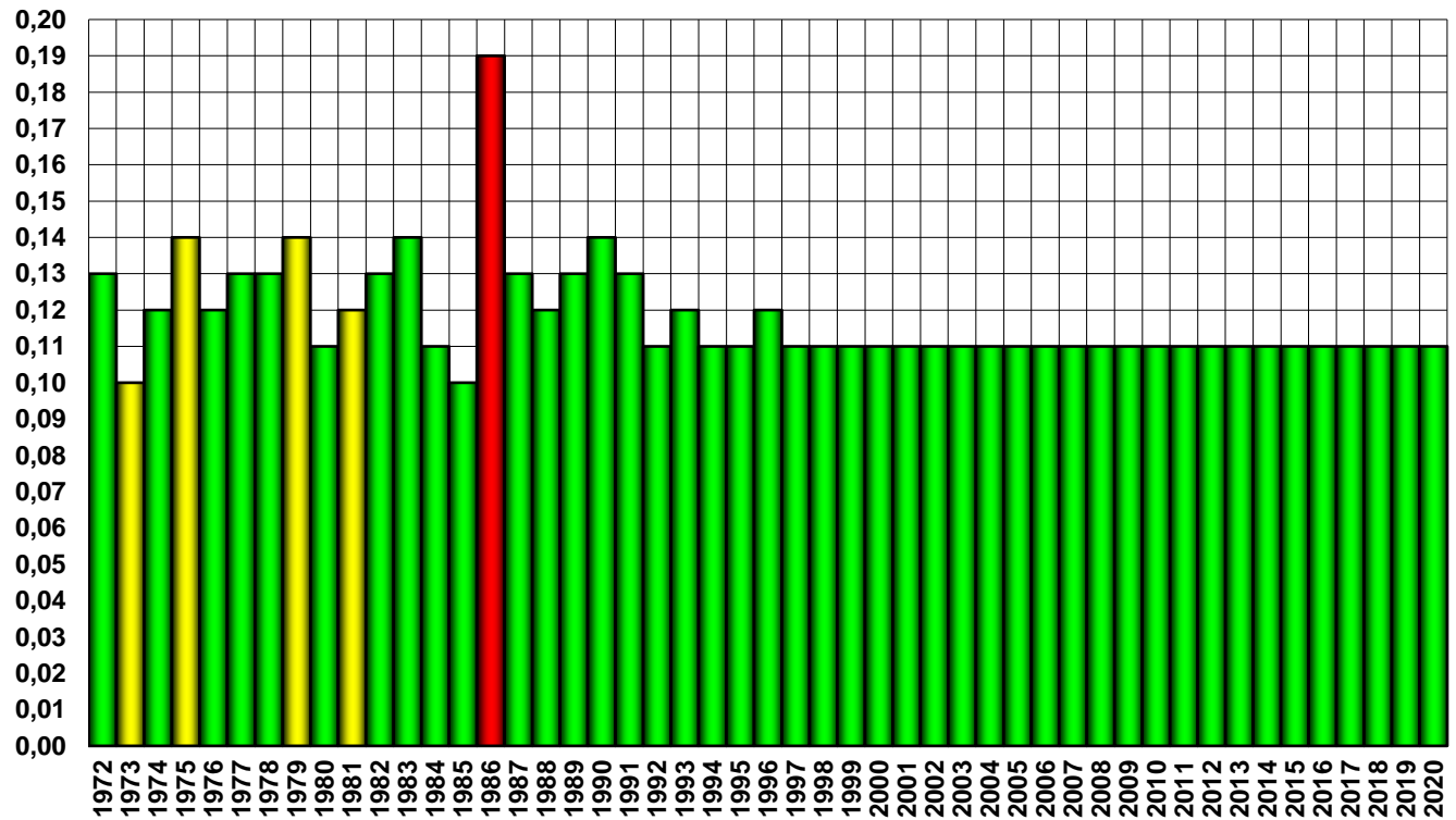
Рис.6.3.2.5. Мощность дозы в районе расположения Ленинградской АЭС, мкЗв/час
