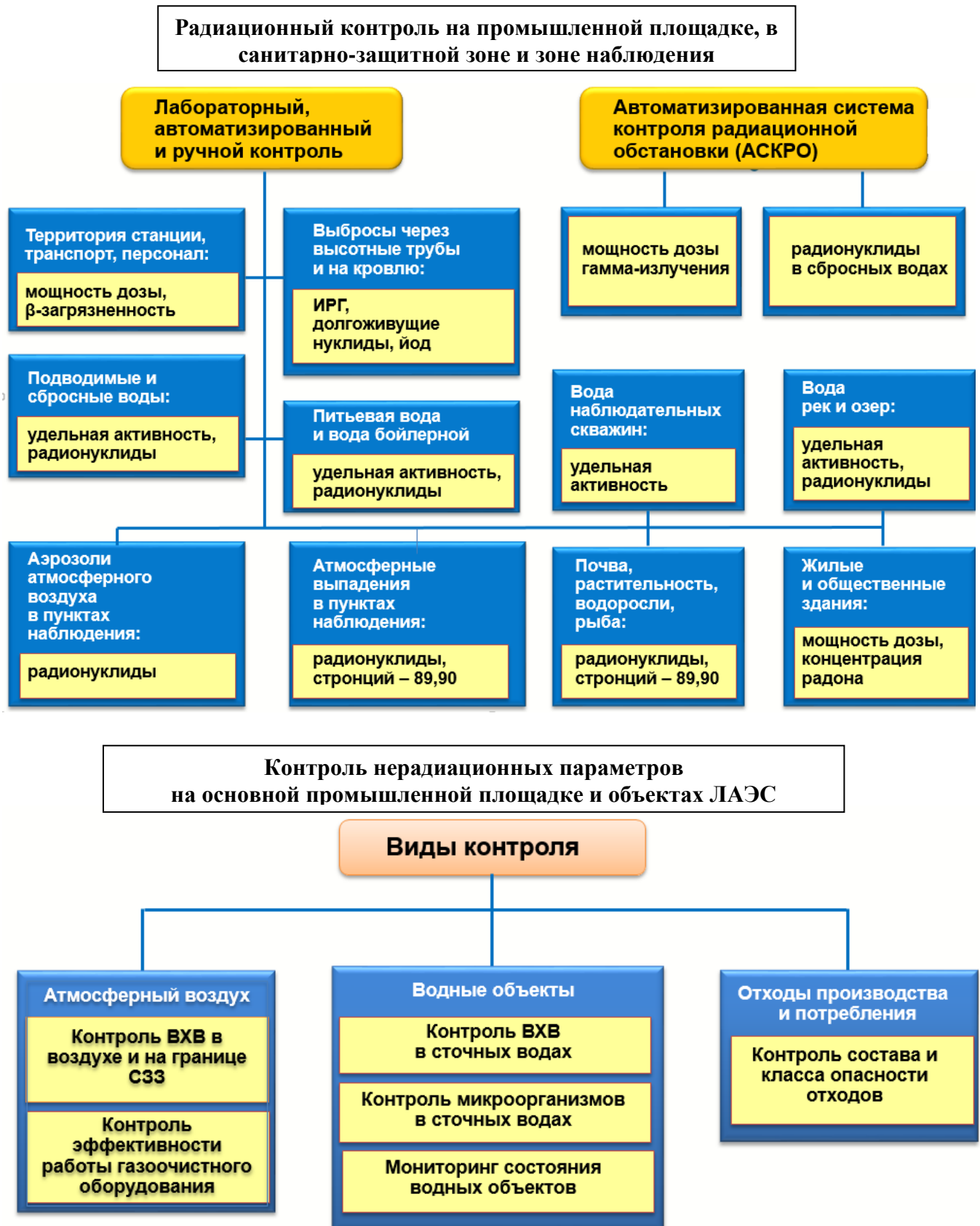
Рис. 5.2. Виды производственного экологического контроля на Ленинградской АЭС
