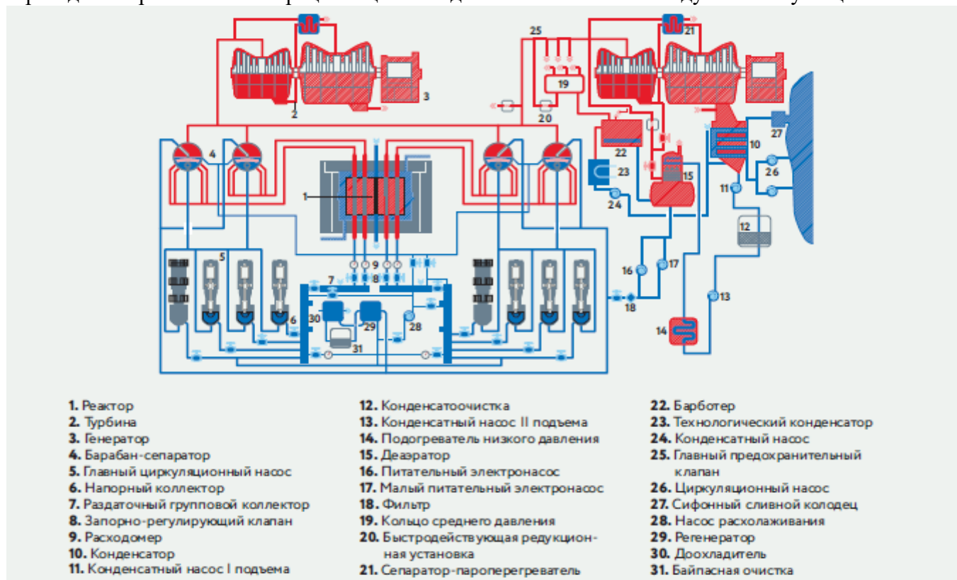
Рис. 1.2 – Принципиальная схема энергоблока РБМК-1 000
