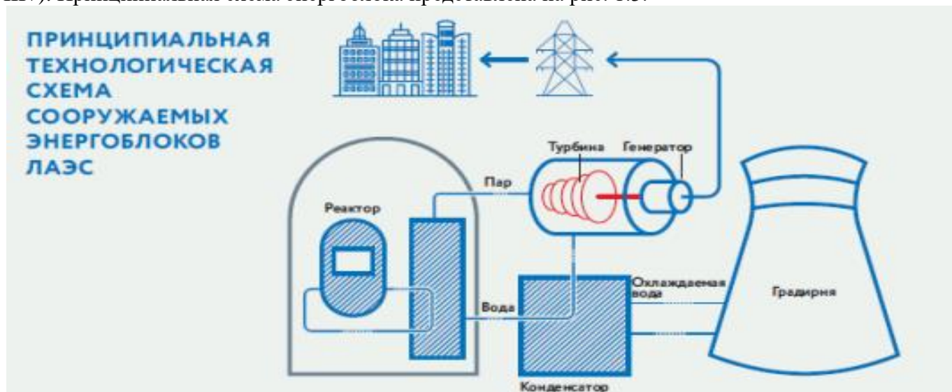
Рис. 1.3 – Принципиальная схема энергоблока ВВЭР-1 200
