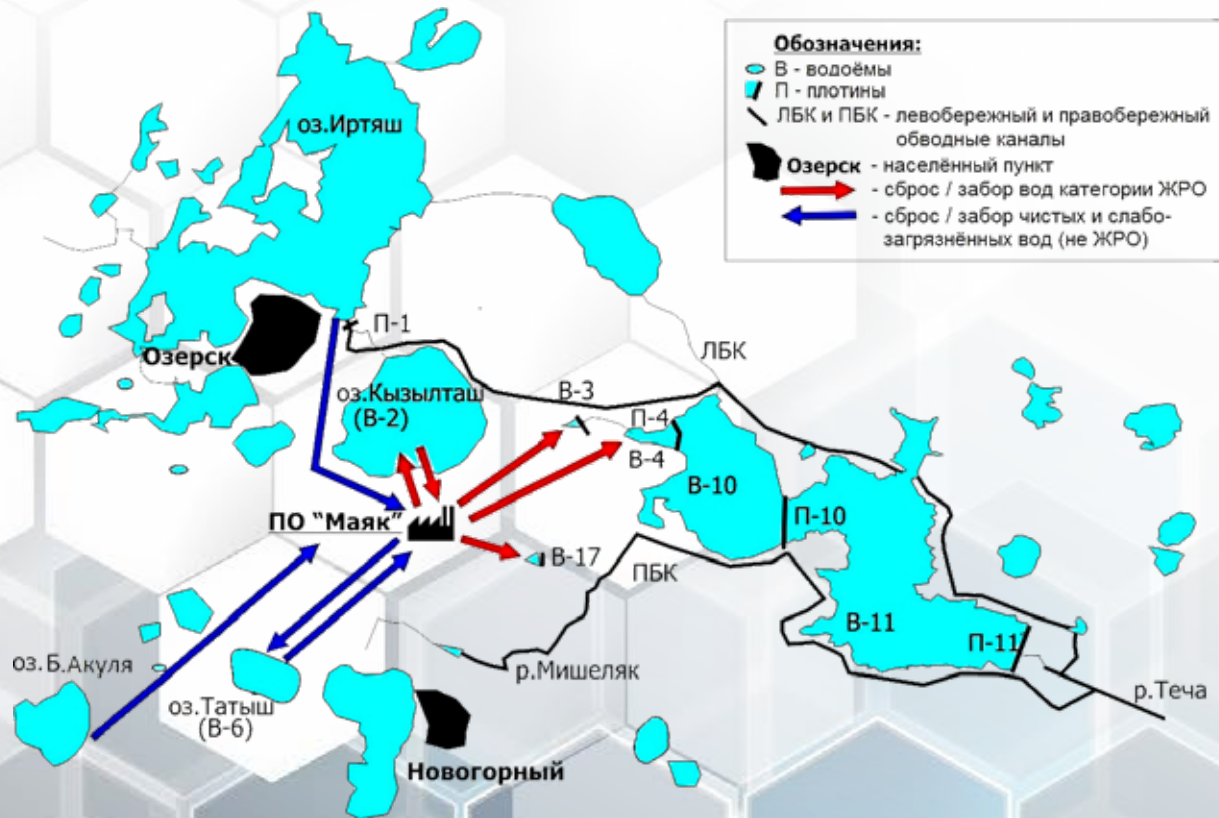
Схема водопользования ФГУП «ПО «Маяк»
